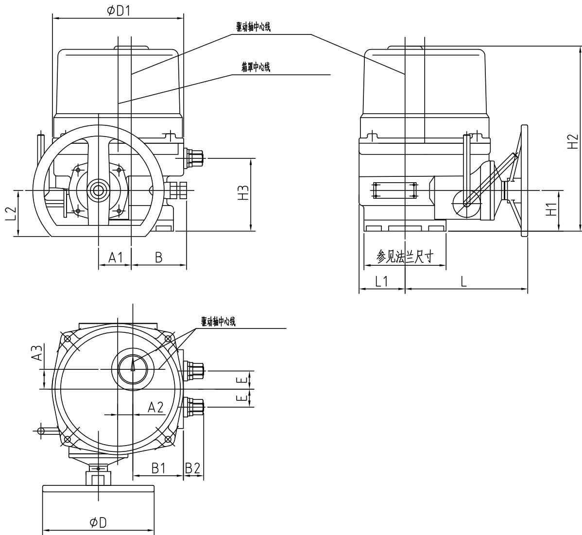
QT1~QT4系列外形尺寸
